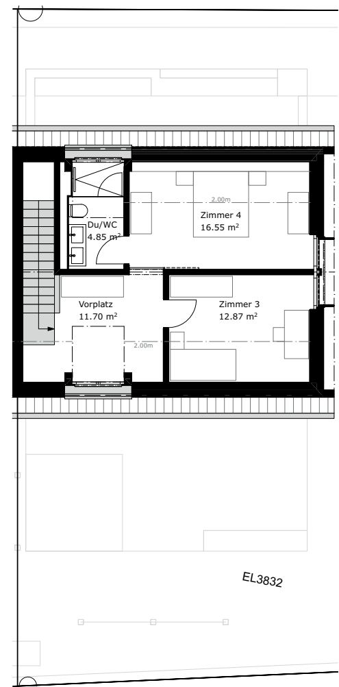
Dachgeschoss
